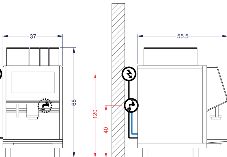
Vista Elevación
